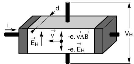
fig. 21 : schéma théorique du capteur à effet Hall.
