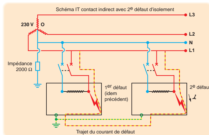
Schéma IT avec un 2 ème défaut d'isolement
