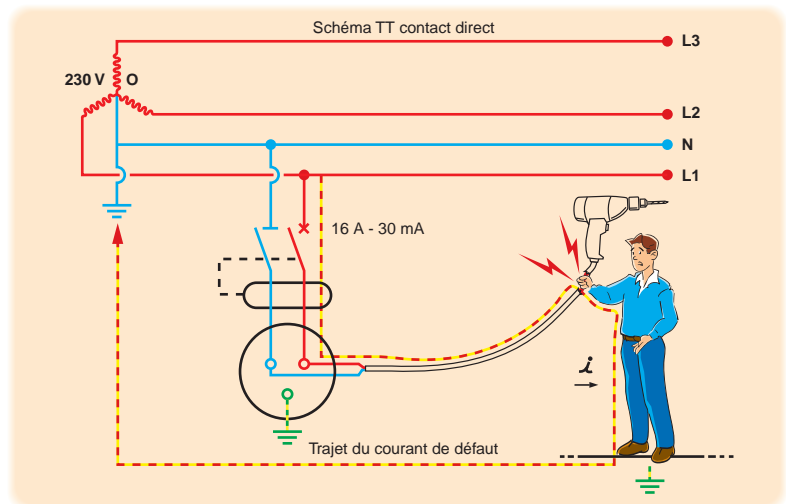
Schéma TT
