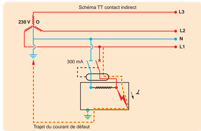
Schéma TT
