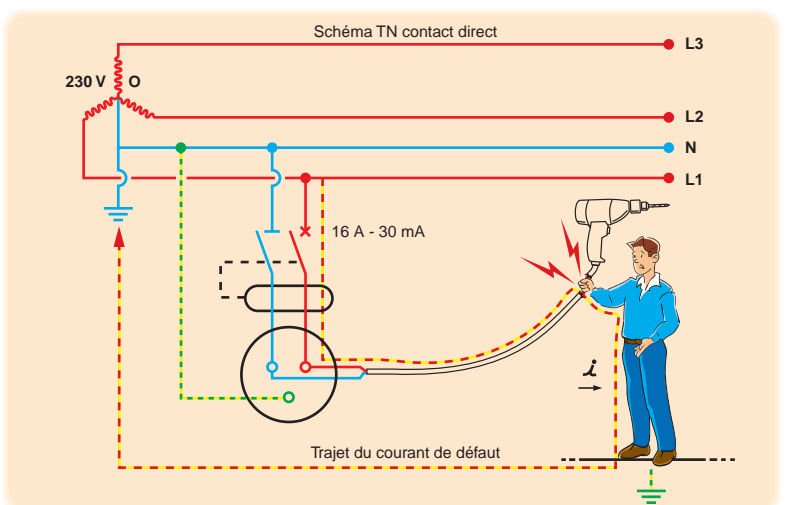
Schéma TN
