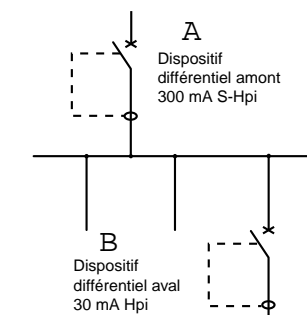
Exemple de sélectivité à 2 niveaux
