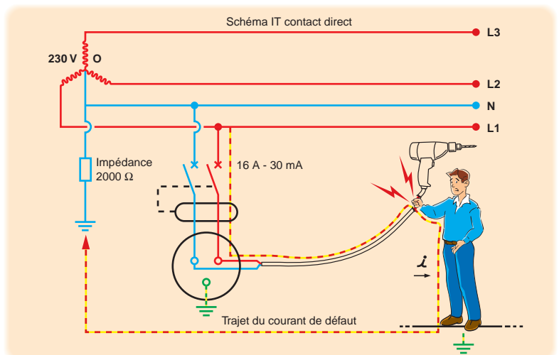
Schéma IT
