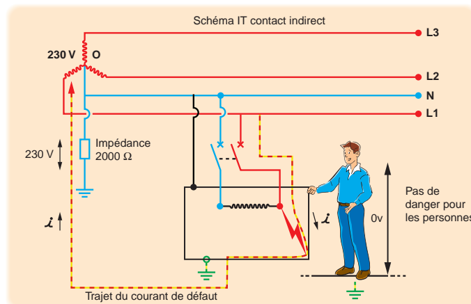
Schéma IT avec un 1 er défaut d'isolement
