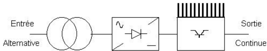
Fig. 7 : Alimentation linéaire
