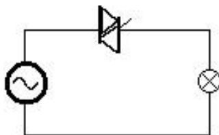
Fig. 12 : Utilisation d'un gradateur
