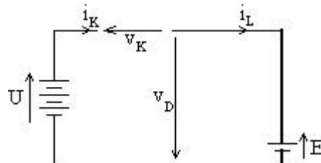
Fig. 19 : Schéma partiel de fonctionnement pour D et K bloqués
