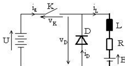
Fig. 16 : Hacheur dévolteur sur charge R, L, E.
