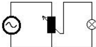
Fig. 11 : Gradation par autotransformateur
