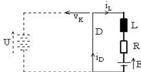
Fig. 18 : Schéma partiel de fonctionnement pour D conductrice et K bloqué
