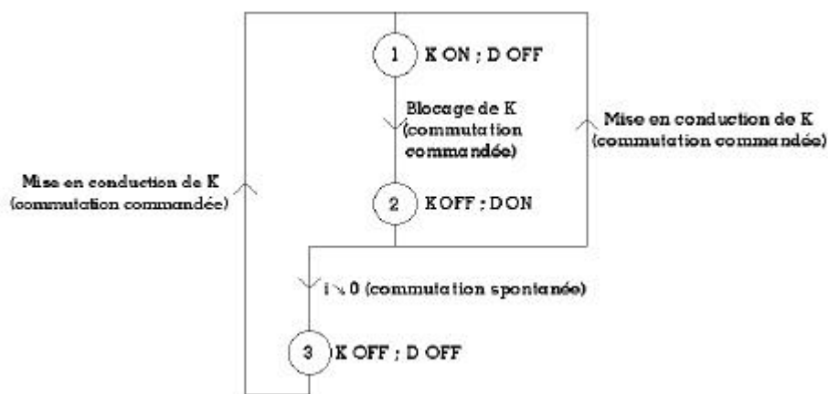
Fig. 20 : Séquences de fonctionnement du hacheur dévolteur
