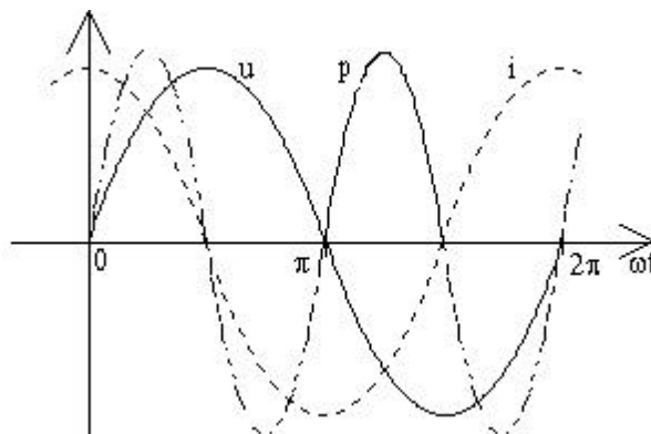
Fig. 15 : Tension, courant et puissance instantanée relatifs à un condensateur alimenté par une tension sinusoïdale.
