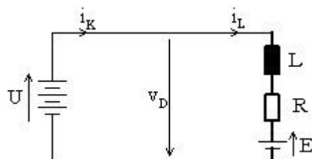
Fig. 17 : Schéma partiel de fonctionnement pour K conducteur et D bloquée
